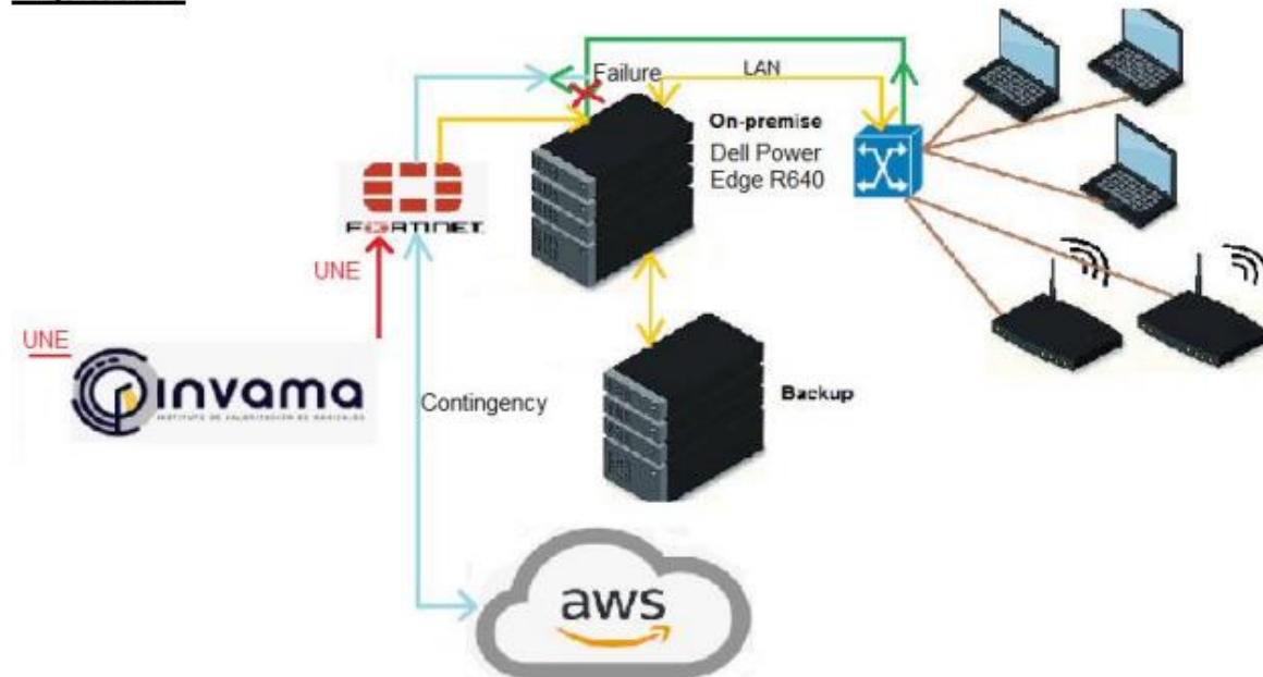
Ilustración 29. Esquema renovación tecnológica Data Center
